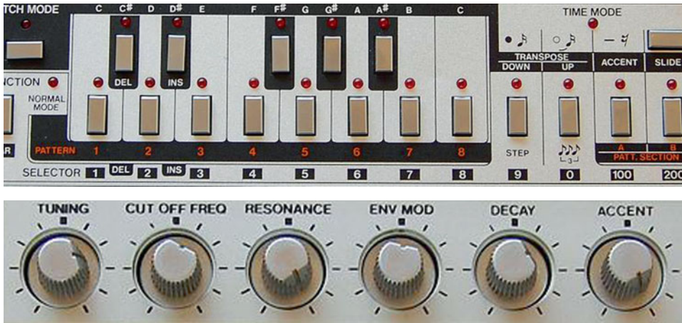
Bild 4: Klaviatur und Parameterpanel der TB-303
